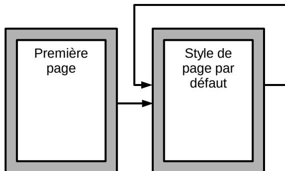
Figure 14 : Flux des styles de pages
